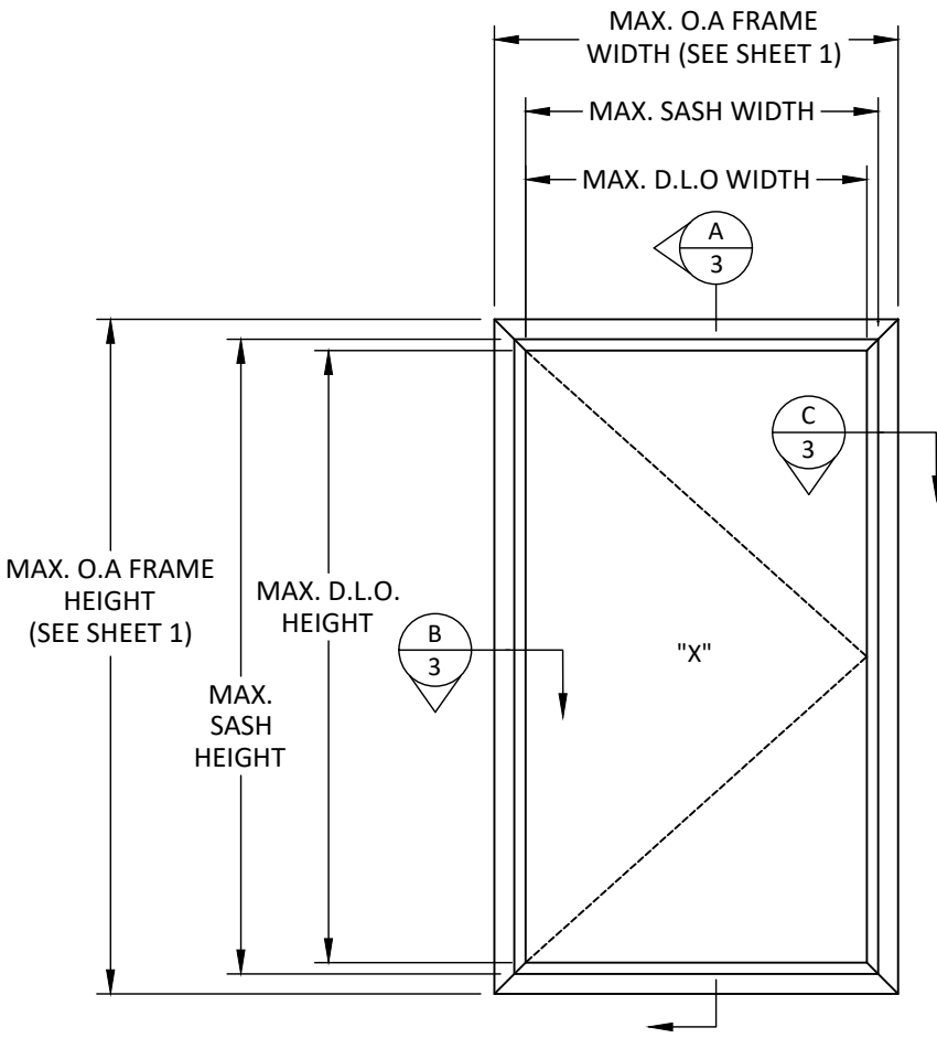
ELEVATION BALCONY DOOR
